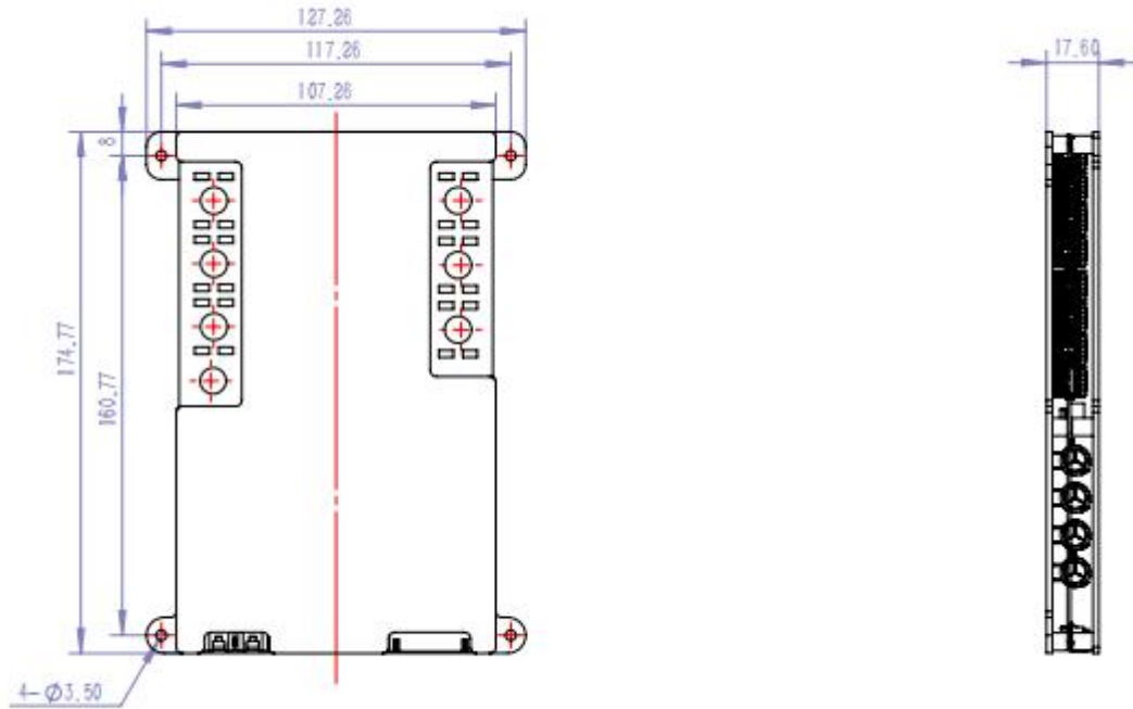
JK-B2A8S-30P 外形尺寸
