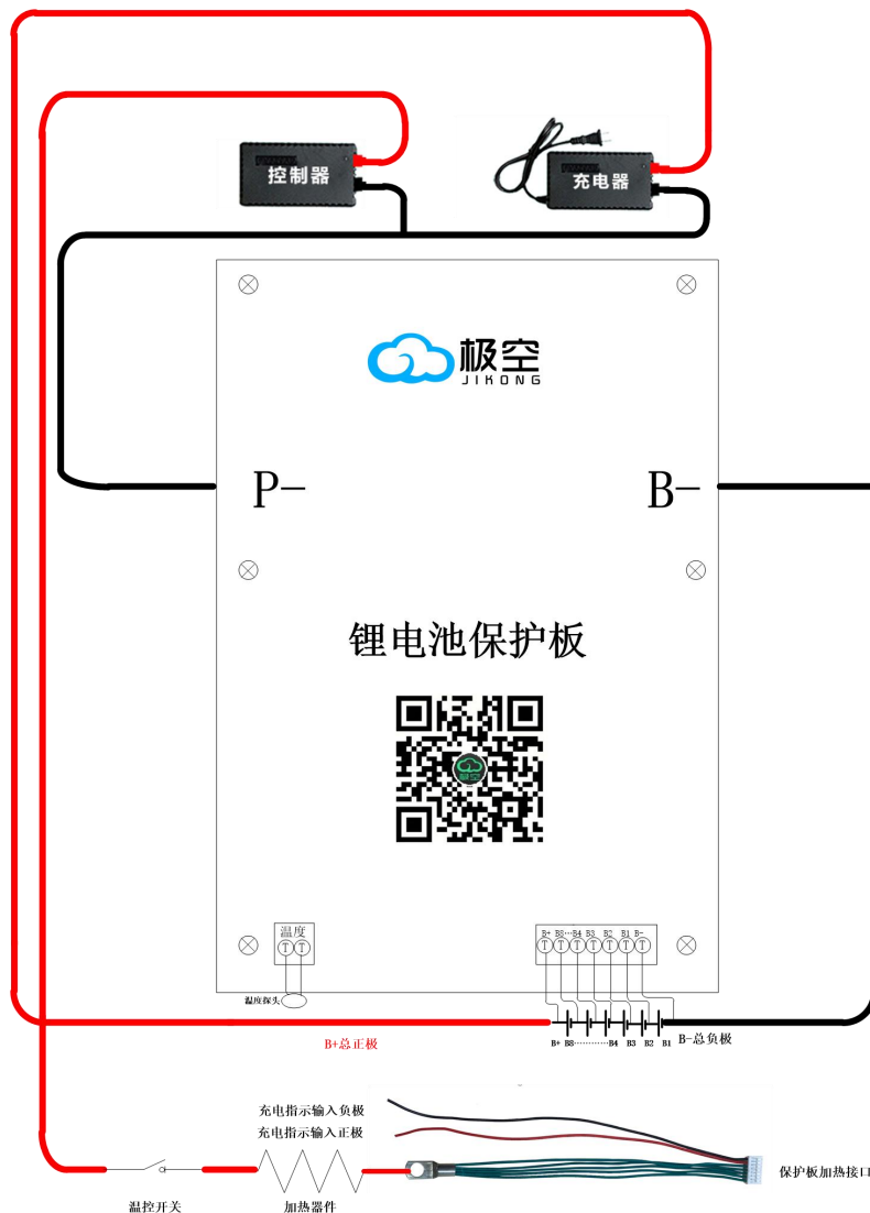
JK-B2A8S-30P接线图
